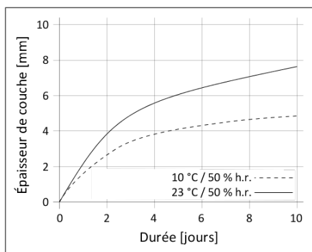
Diagramme 1: Vitesse de durcissement de Sikaflex®-529 Evolution
