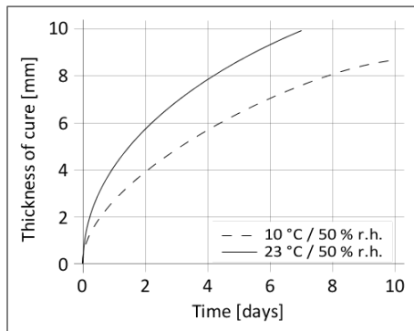
Diagram 1: Vitesse de polymérisation du Sikaflex®-290 DC PRO
