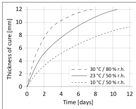
Diagram 1: Rychlost vytvrzení Sikaflex®-821 FR
