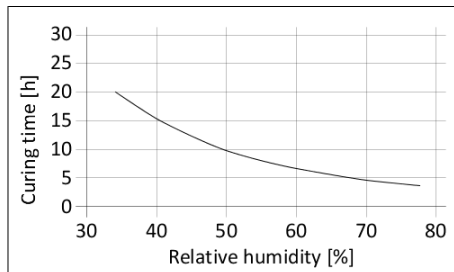
Diagram 1: Doba vytvrzení pro tloušťku filmu 500 µm
