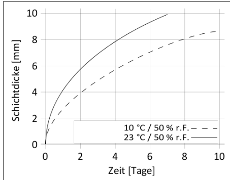
Diagramm 1: Durchhärtegeschwindigkeit SikaTack® PRO (Purform®)
