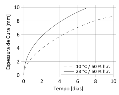
Diagrama 1: Velocidade de cura de Sikaflex®-290 DC PRO
