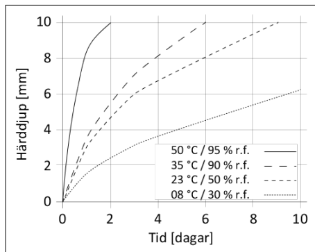
Diagram 1: Härdningshastighet Sikasil® SG-20
